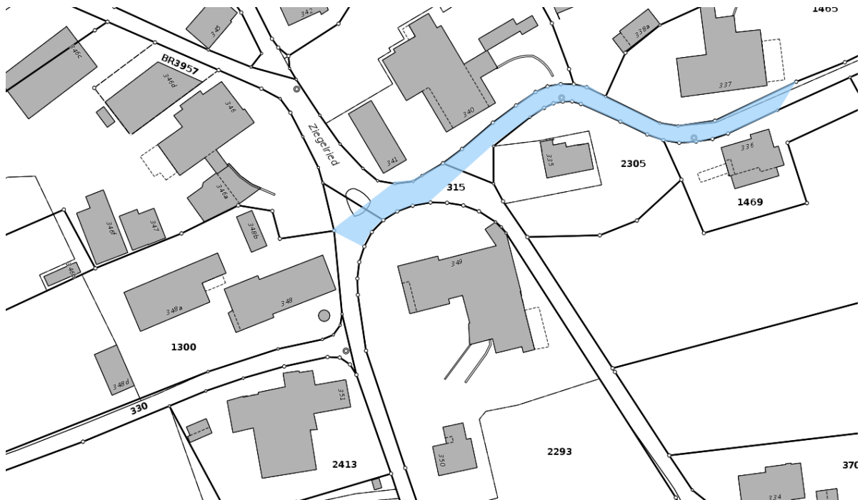
Perimeter Wasserleitungersatz
